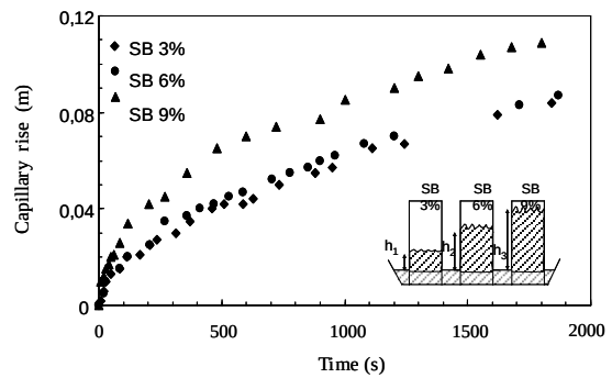
Fig. 7 Capillary rise. Soil/Bentonite
